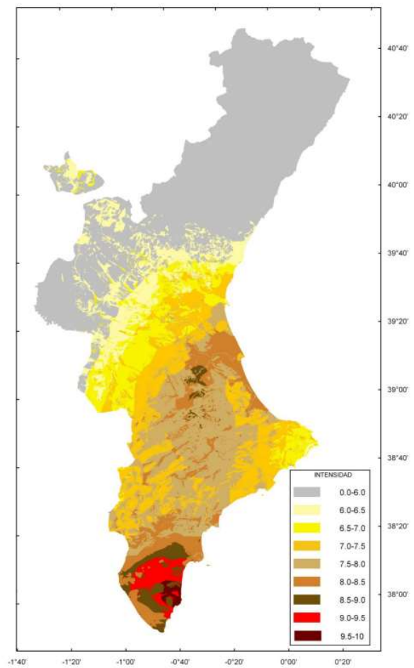
MAPA DE INTENSIDAD SÍSMICA (PERIODO DE RETORNO 1000 AÑOS)
