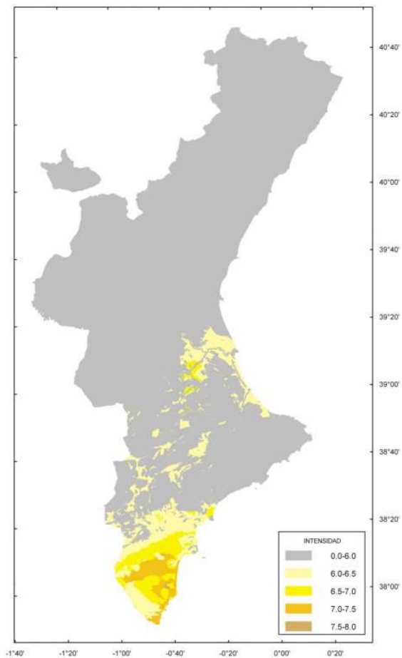
MAPA DE INTENSIDAD SÍSMICA (PERIODO DE RETORNO 100 AÑOS)
